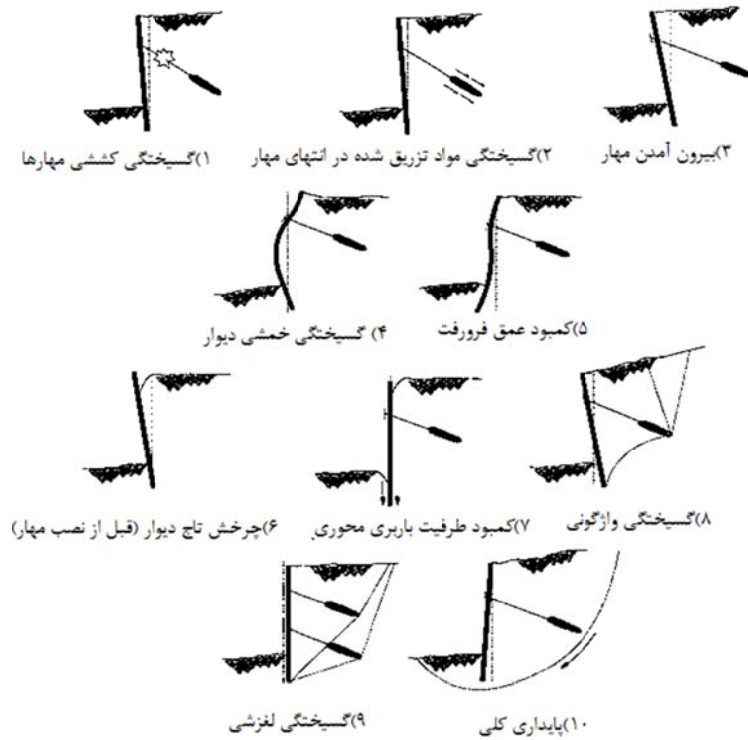
شکل ۷-۵-۱-۵-۷ حالت‌های حدی دیوارهای مهار شده
