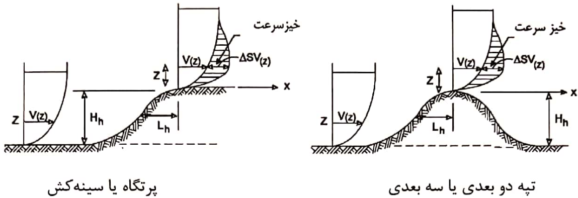
شکل ۶-۱۰-۱ افزایش سرعت باد در بالای تپه‌ها و پرتگاه‌ها
