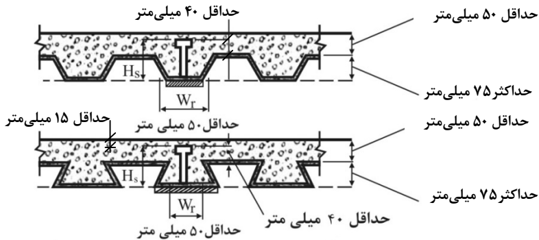
شکل ۲-۱۰-۲-۴ ملاحظات و محدودیت‌های ورق‌های فولادی شکل داده شده
