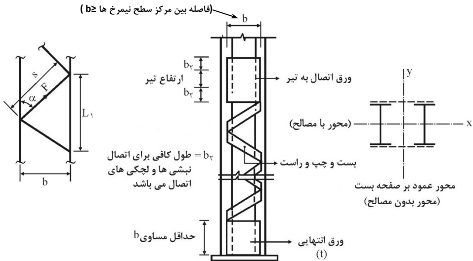
شکل ۱۰-۲-۴-۳ عضو فشاری ساخته شده با بست‌های مورب
