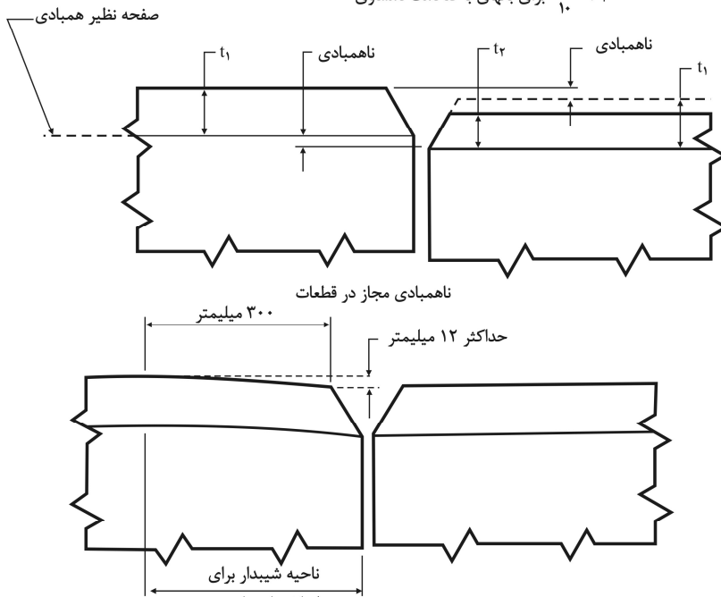
شکل ۴-۱۰-۲ اصلاح ناهمبادی و ناهم‌محوری
