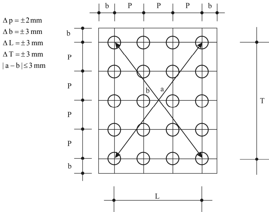
شکل ۱۰-۴-۱۲ رواداری سوراخ‌های پیچ
