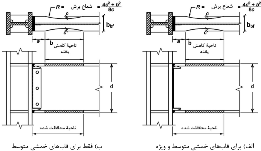
شکل ۱۰-۳-۱۳-۱ اتصال گیردار مستقیم تیر با مقطع کاهش یافته (RBS)
