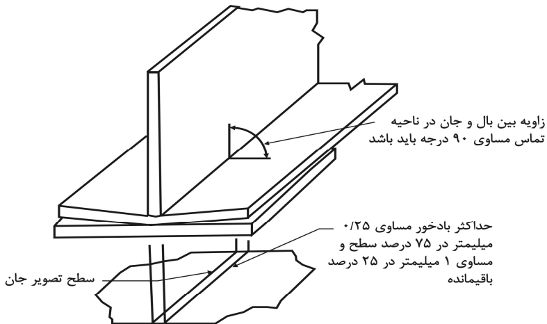
شکل ۱۰-۴-۷ رواداری در محل تماس تیر با تکیه‌گاه - تیر بدون سخت‌کننده تکیه‌گاهی
